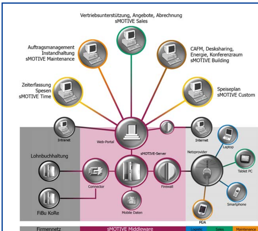
Bild: Systemkonzept der sMOTIVE Middleware
